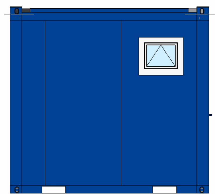
5 Ansicht von Links 1 : 30
