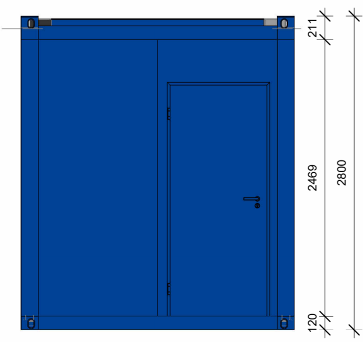
4 Ansicht von Vorne 1 : 30
