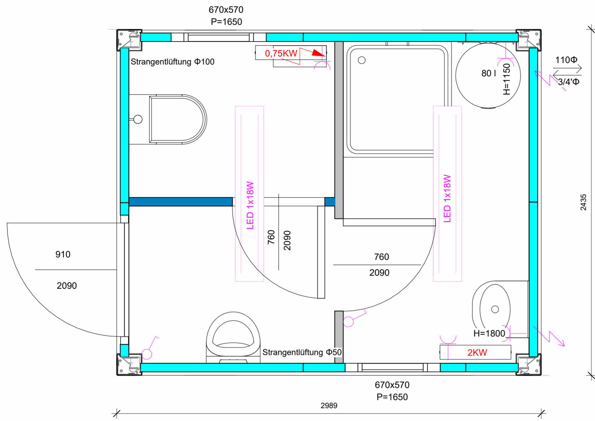
1 Grundriss 1 : 15
