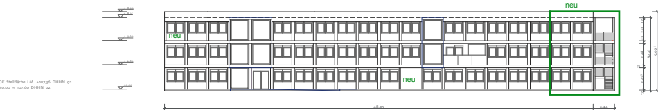
Ansicht Ost
